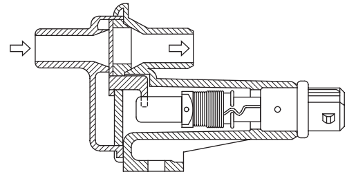
エアレギュレーター
