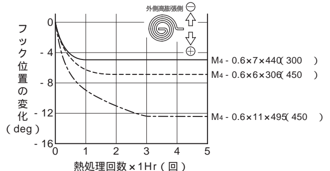
熱処理回数とフック位置の変化
